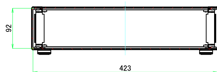
A-A (1:5)
